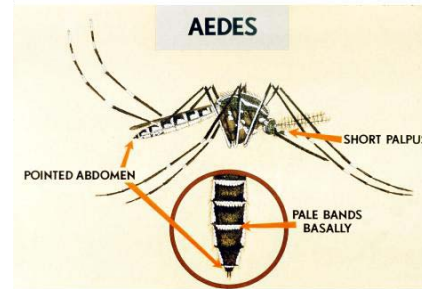
5B. Aedes spp Ochlerotatus spp.
